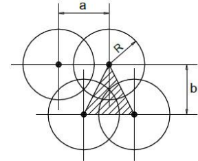
a) Sơ đồ bố trí kiểu tam giác
